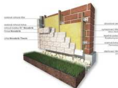
Skladba fasádního pláště tepelně-izolační fasády Novabrik Therm
